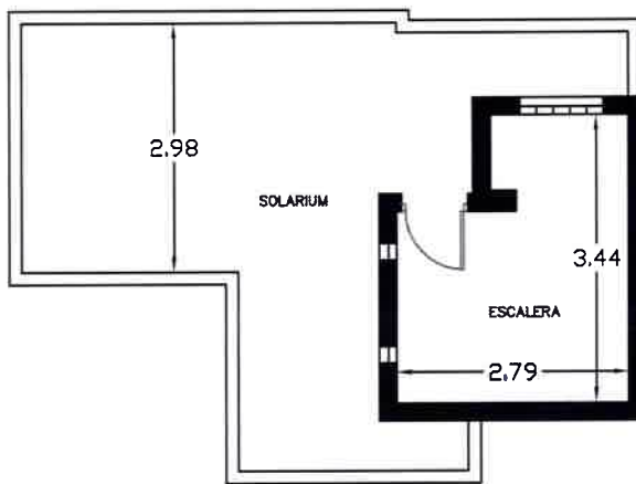
PLANTA CUBIERTA
